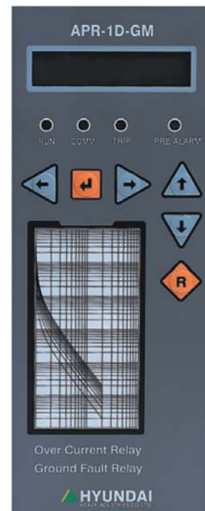
● Рис. 8. Реле защиты воздушного автоматического выключателя. Модель APR-1D-GM
