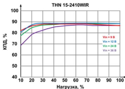
Рис. 5. Зависимость КПД от уровня нагрузки на примере THN 15-2410WIR [5]
