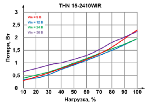
Рис. 7. Уровень потерь на примере THN 15-2410WIR [5]
