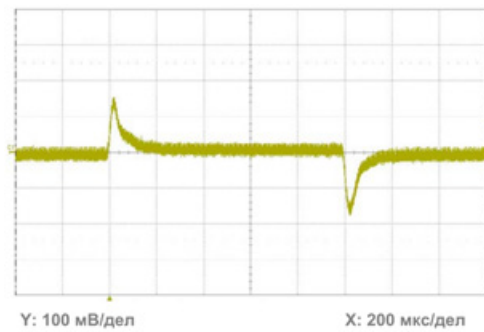
Рис. 3. Отклик на импульсное изменение нагрузки (25%) на примере THN 15-2410WIR [5]
