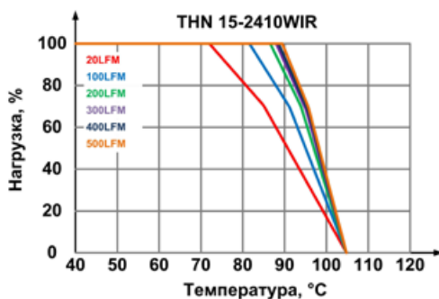
Рис. 8. Ограничение выходной мощности на примере THN 15-2410WIR [5]
