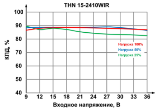
Рис. 6. Зависимость КПД от входного напряжения на примере THN 15-2410WIR [5]
